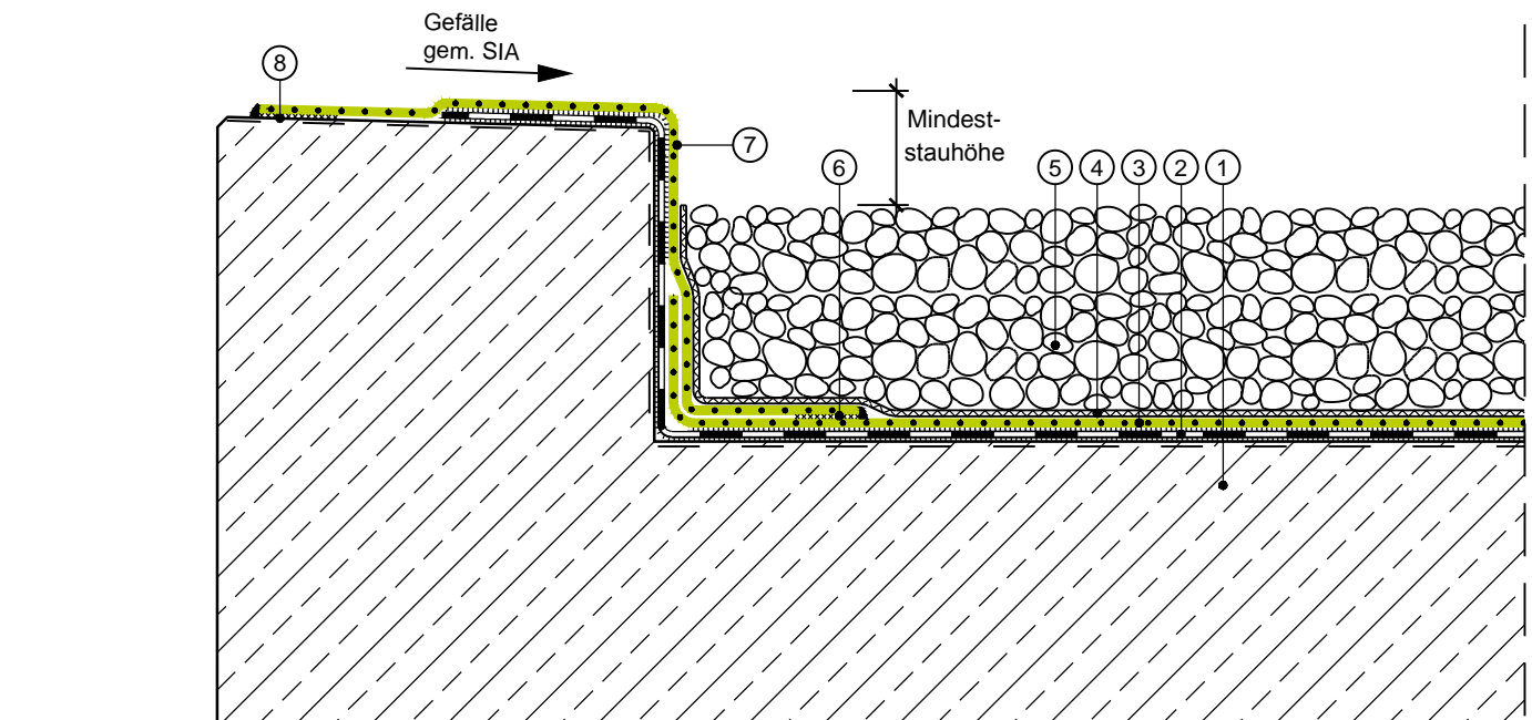
Maßstab 1:5 (Abdichtungsbahnen sind überhöht dargestellt)
